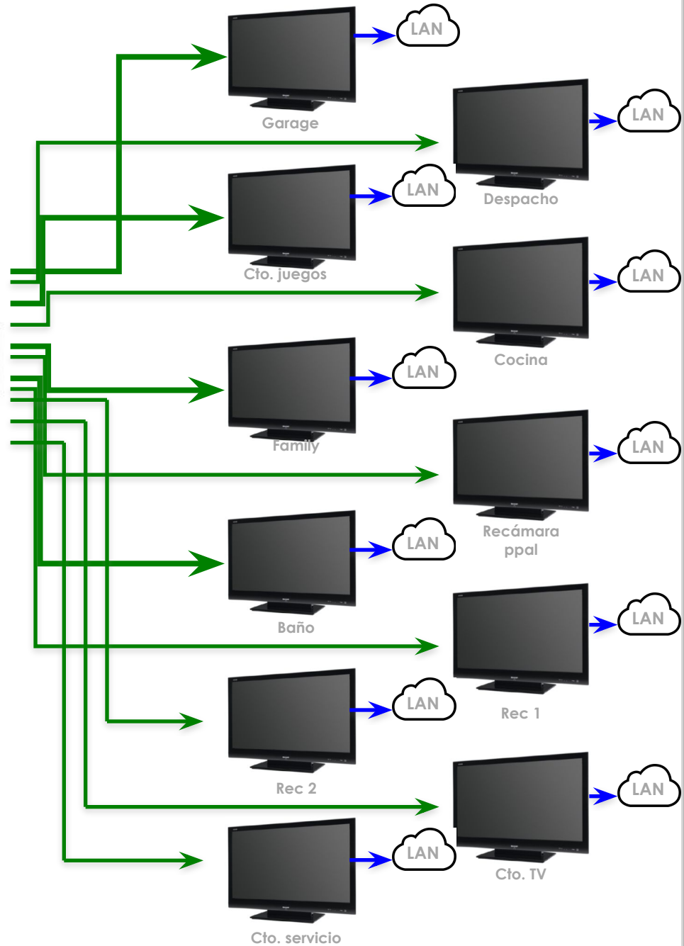
DISTRIBUIDOR RF MONTADO EN RACK
